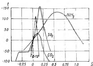
Hình 1-1. Đường cong giới hạn pha của một số loại tác nhân lạnh \text{NH}_3 , \text{SO}_2 , \text{CO}_2 , F-12.
