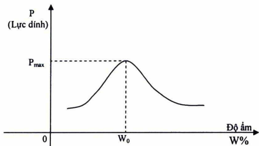
Hình 1.1: Sự phụ thuộc của P - lực bêtt dính và độ ẩm w
