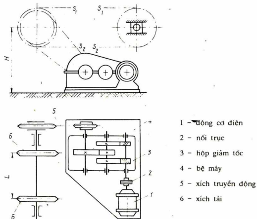
Hình 1.1. Sơ đồ hệ dẫn động xích tải
