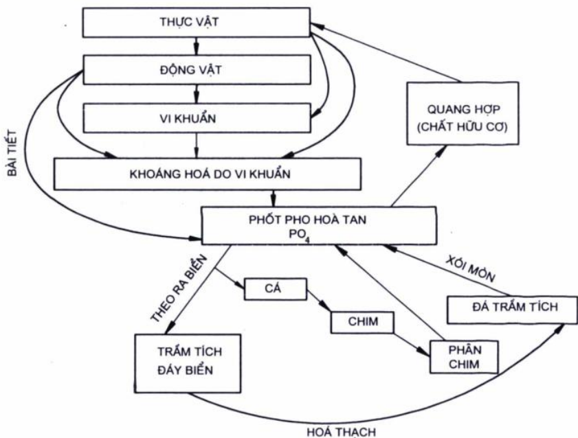
Hình 1-3. Vòng tuần hoàn photpho.
