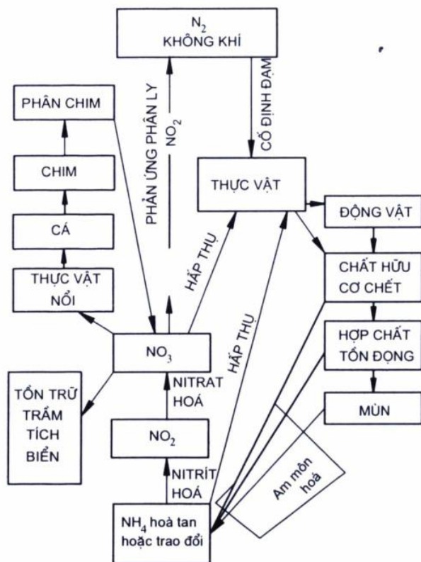
Hình 1-4. Vòng tuần hoàn nitơ.
