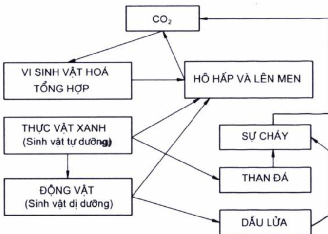
Hình 1-2. Vòng tuần hoàn các bon.
