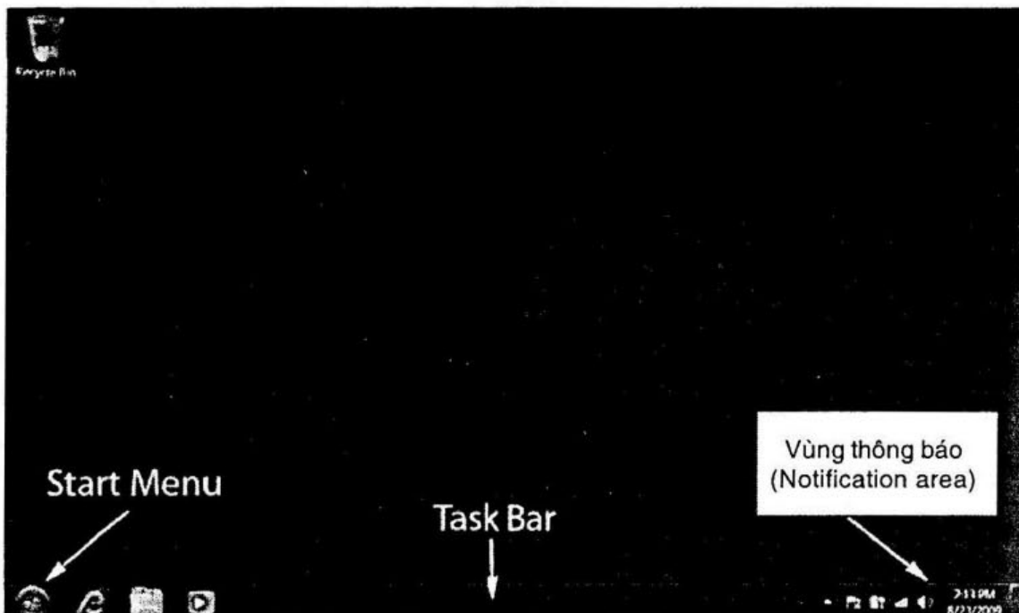
Hình 1.1 Desktop Windows 7
