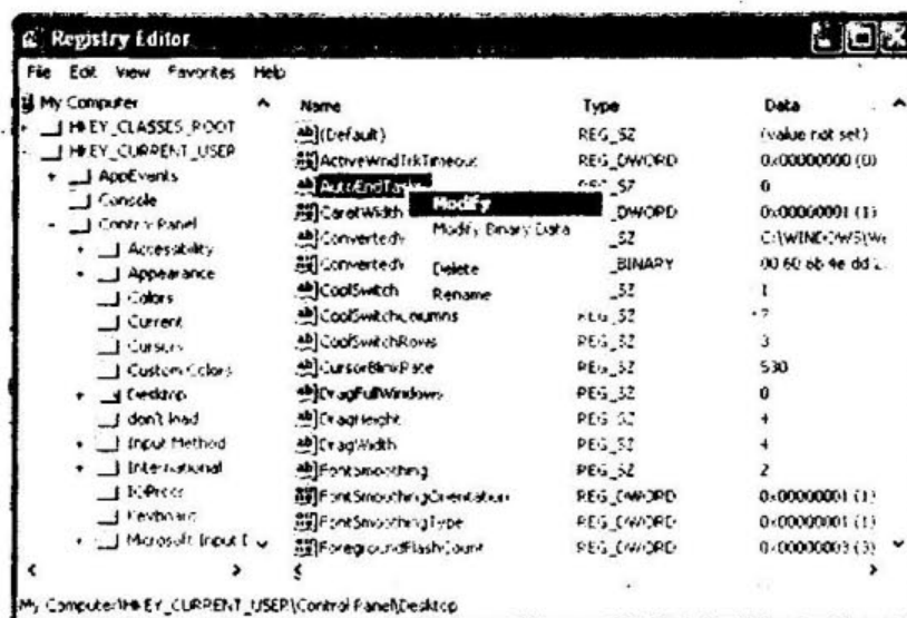
Hình 3. Cửa sổ Registry Editor
