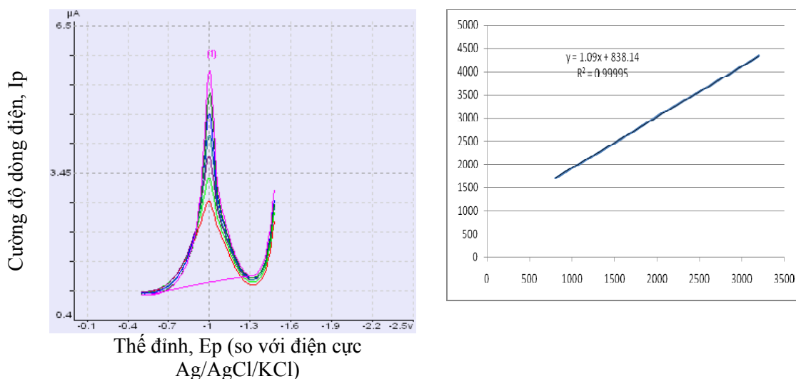
Hình 3. Đường chuẩn của DI ghi trong điều kiện đã xác định (AdSWSV, dung dịch nền amoni acetat 0,4 N pH 4,3, V_{\text{pulse}} 40 mV, V_{\text{step}} 10 mV, T_{\text{drop}} 5 giây, T_c 6 giây và V_c -500 mV).
