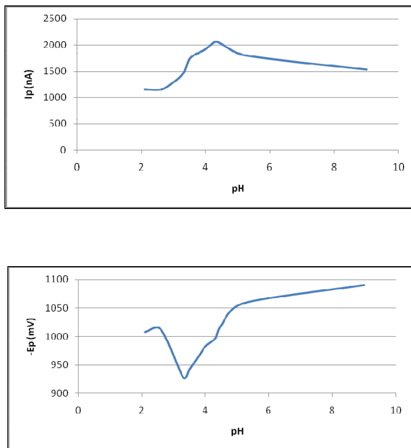
Hình 1. Ảnh hưởng của pH trên sóng phổ của DI trong dung dịch nền amoni acetat 0,1 N, biên độ xung 30 mV, bước thế 8 mV, thời điểm bắt đầu quét thế 4 giây.
