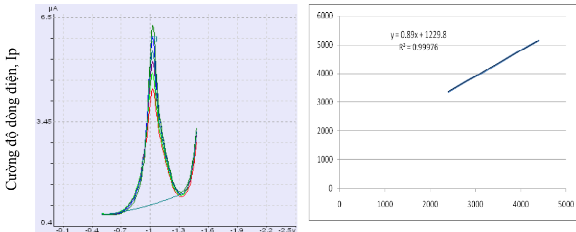
Hình 4. Đường chuẩn của DI ghi nhận khi có bổ sung dịch chiết lá artichoke (AdSWSV, dung dịch nền amoni acetat 0,4 N pH 4,3, V_{\text{pulse}} 40 mV, V_{\text{step}} 10 mV, T_{\text{drop}} 5 giây, T_e 6 giây và V_e -500 mV).
