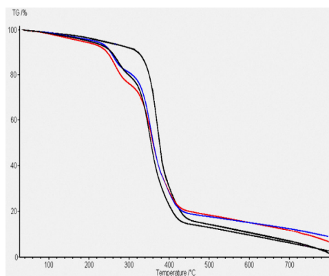
Hình 7. Giải đồ TGA của các composít: (a) TPS/NR/ENR (40/60/15), (b) TPS/NR/ENR (70/30/15), (c) TPS/NR/ENR (80/20/15).
